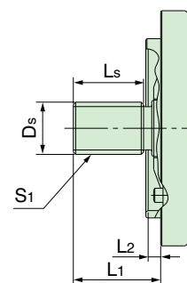
●SAEスプライン入力軸形状 Splined shaft
