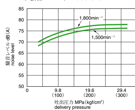
◆ 騒音レベル／Noise level
